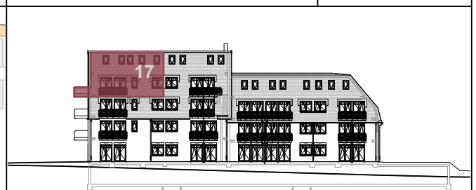
Ansicht WEST
