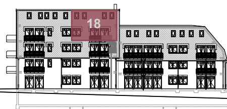
Ansicht WEST
